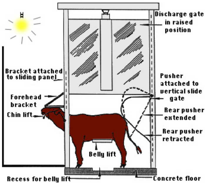
Apparaat voor koosjer slachten, ontworpen door Temple Grandin
